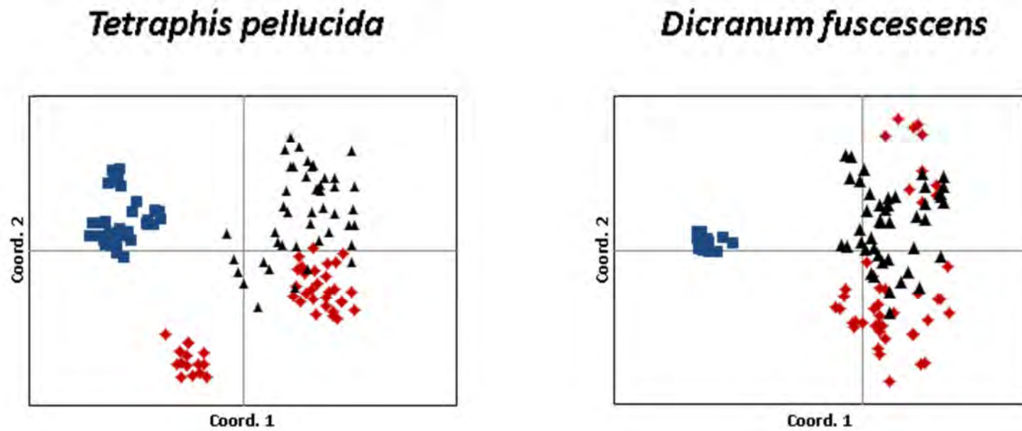
Figure 2.5 Analyse en coordonnées principales à l'échelle des populations des deux espèces Tetraphis pellucida et Dicranum fuscescens (rouge: Population 1 Lebel-sur-Quévillon, bleue: Population 2 La Sarre, noire: Population 3 Lebel-sur-Quévillon).
