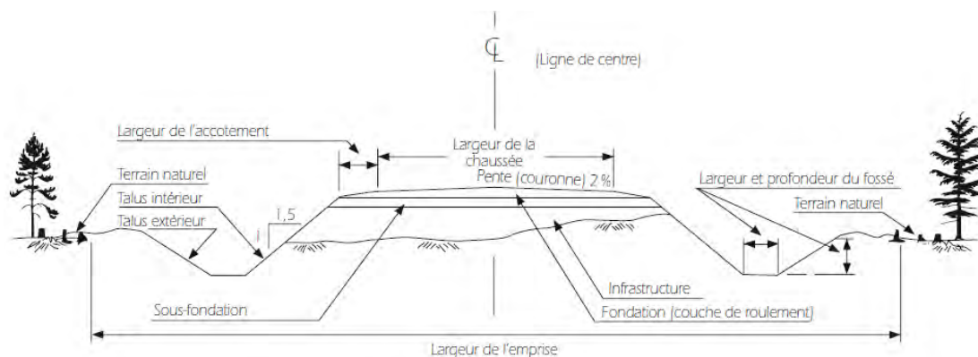
Figure 1.1 Caractéristiques morphologiques d'un chemin forestier (Desautels et al., 2009).
